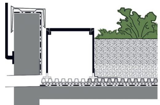
Κατασκευαστική λεπτομέρεια υδρορροής με ειδικό φρεάτιο KS 30-PE
