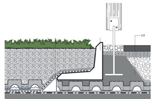
Κατασκευαστική λεπτομέρεια συναρμογής δαπέδου - φύτευσης και στήριξης πέργκολας.
